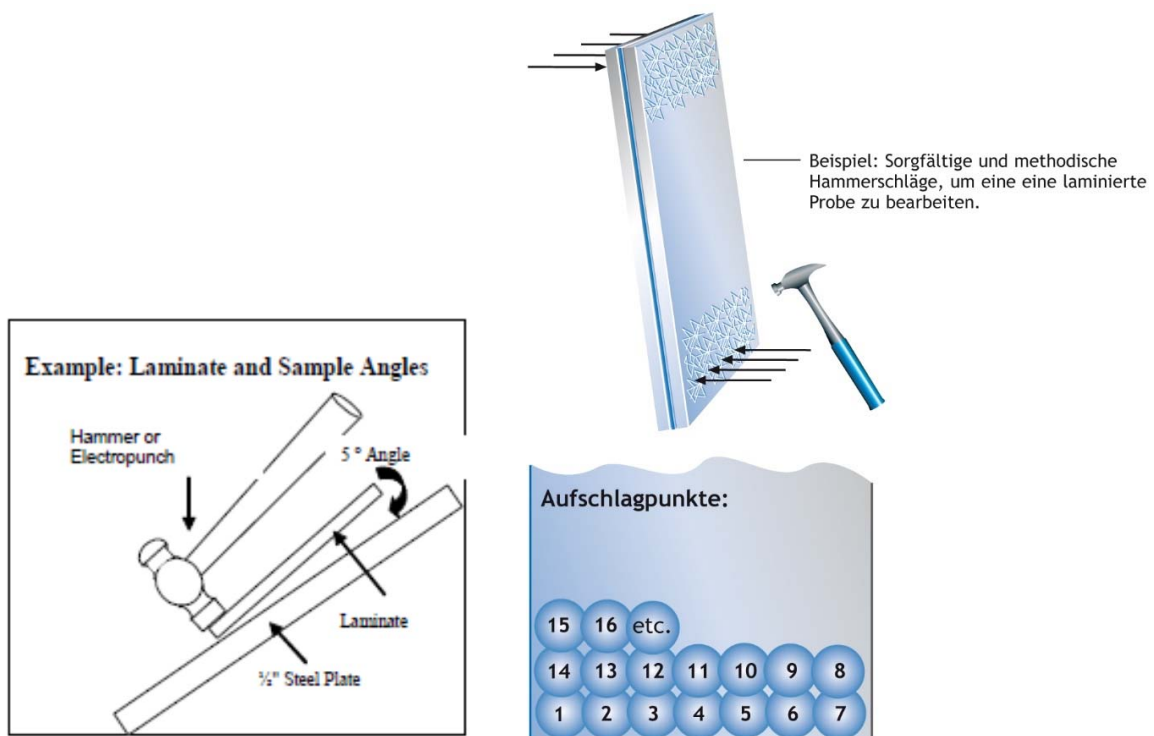
Abb. 3.1: Prüfdurchführung
